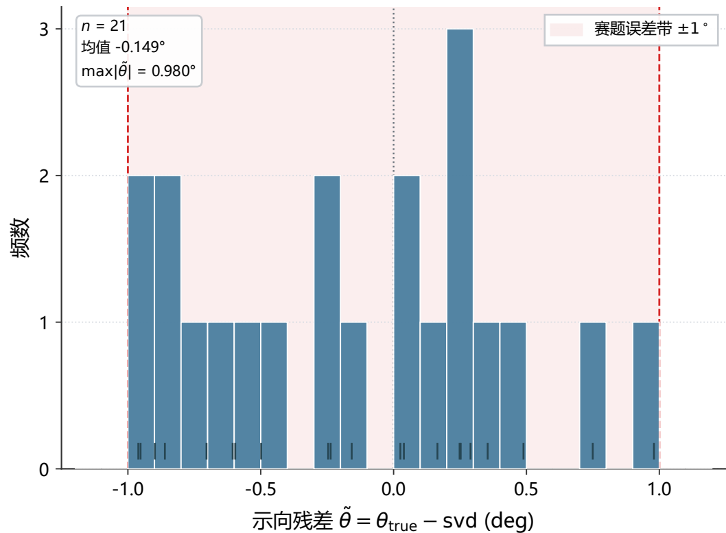
示向残差分布
