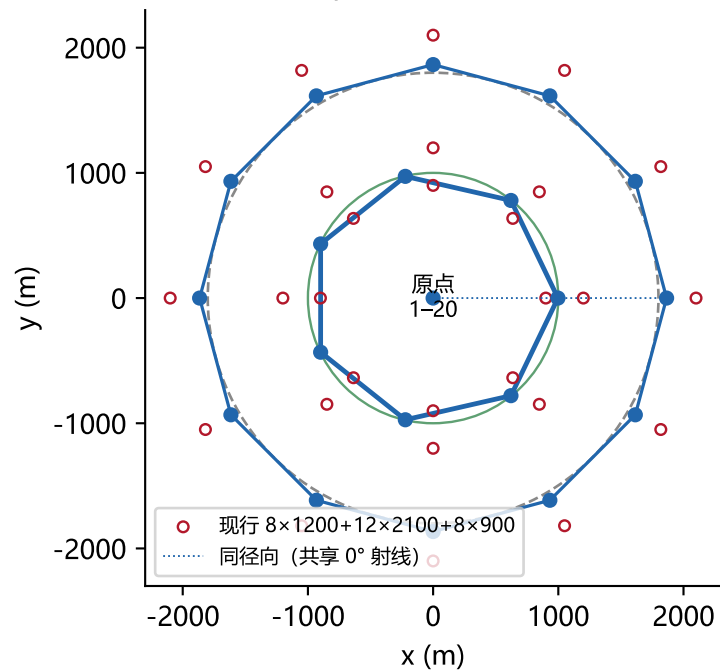
最优：正7边形 \rho=997\text{ m} + 正12边形 1865 m
