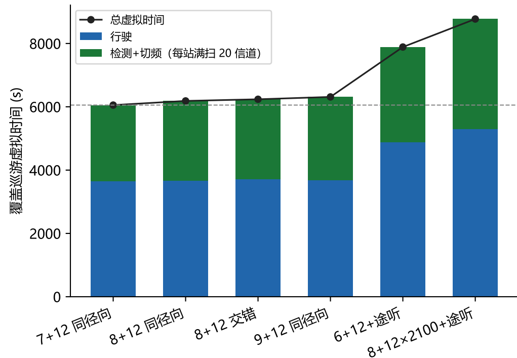
全覆盖（密网格前瓣）下的检测巡游
