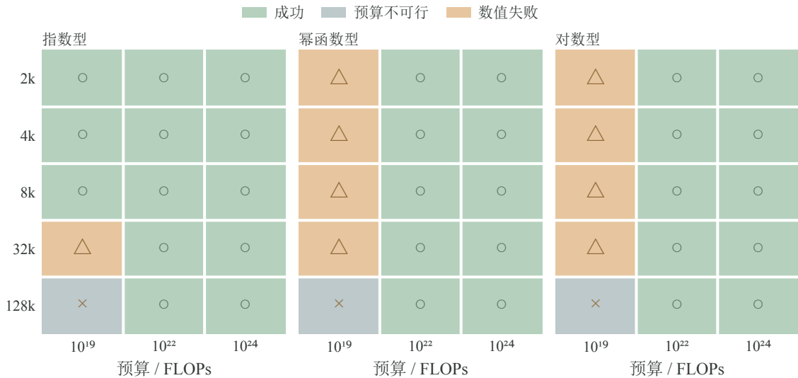
上下文 / Token
