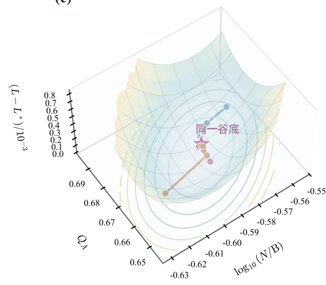
谷底局部放大: 末端汇聚
