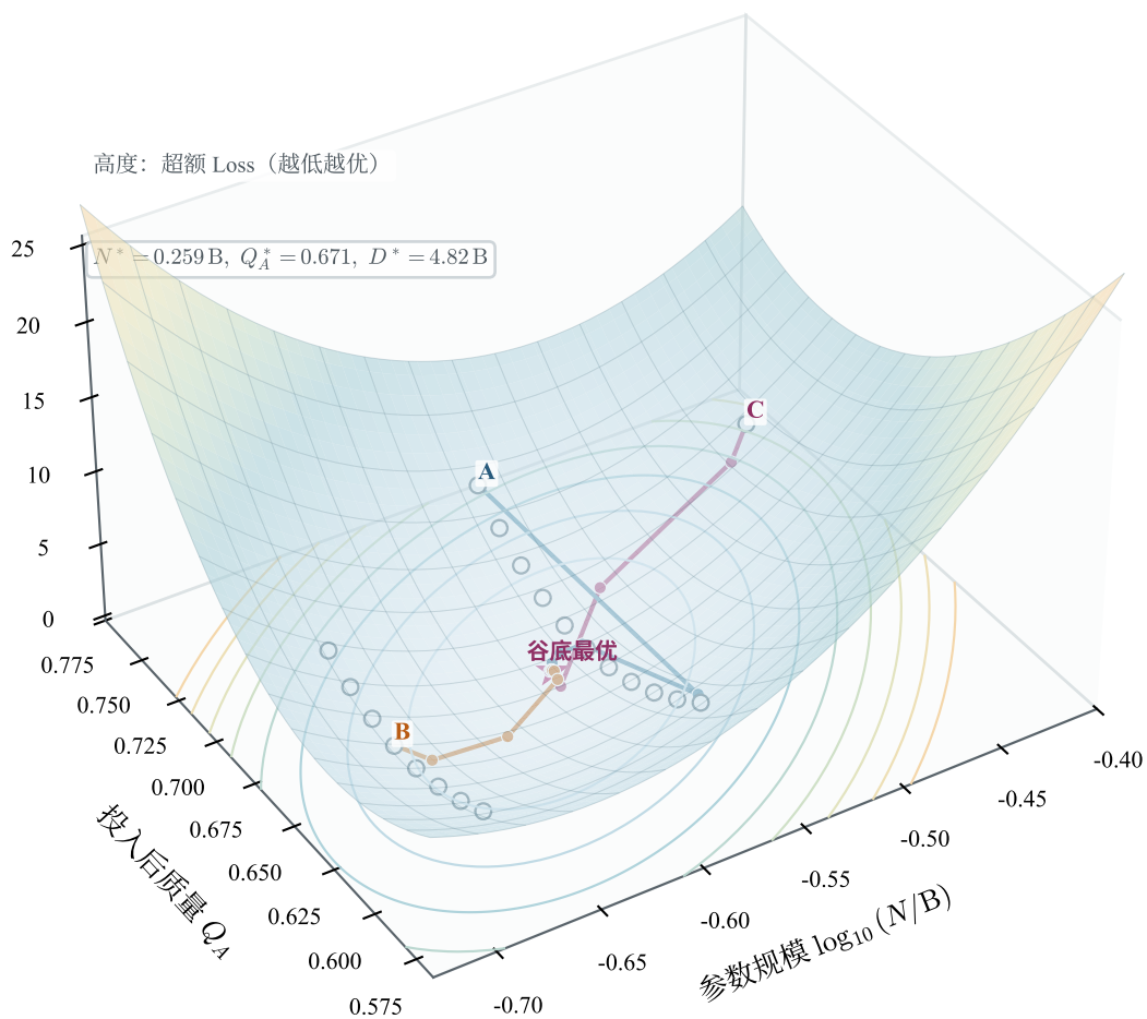
三维 Loss 地形与寻优轨迹
