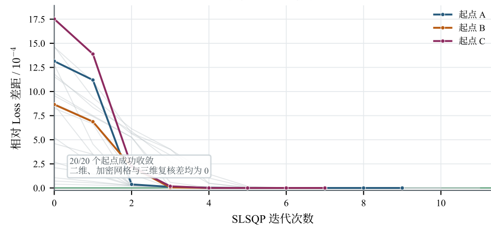
谷底局部放大: 末端汇聚
