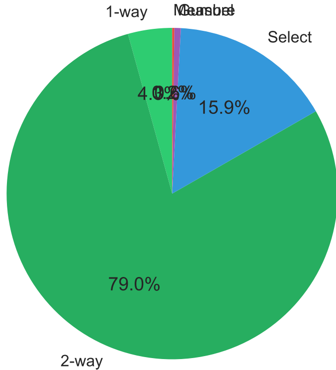
FHAIM-L2
