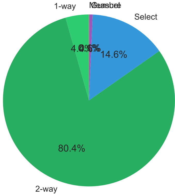
FHAIM-L1
