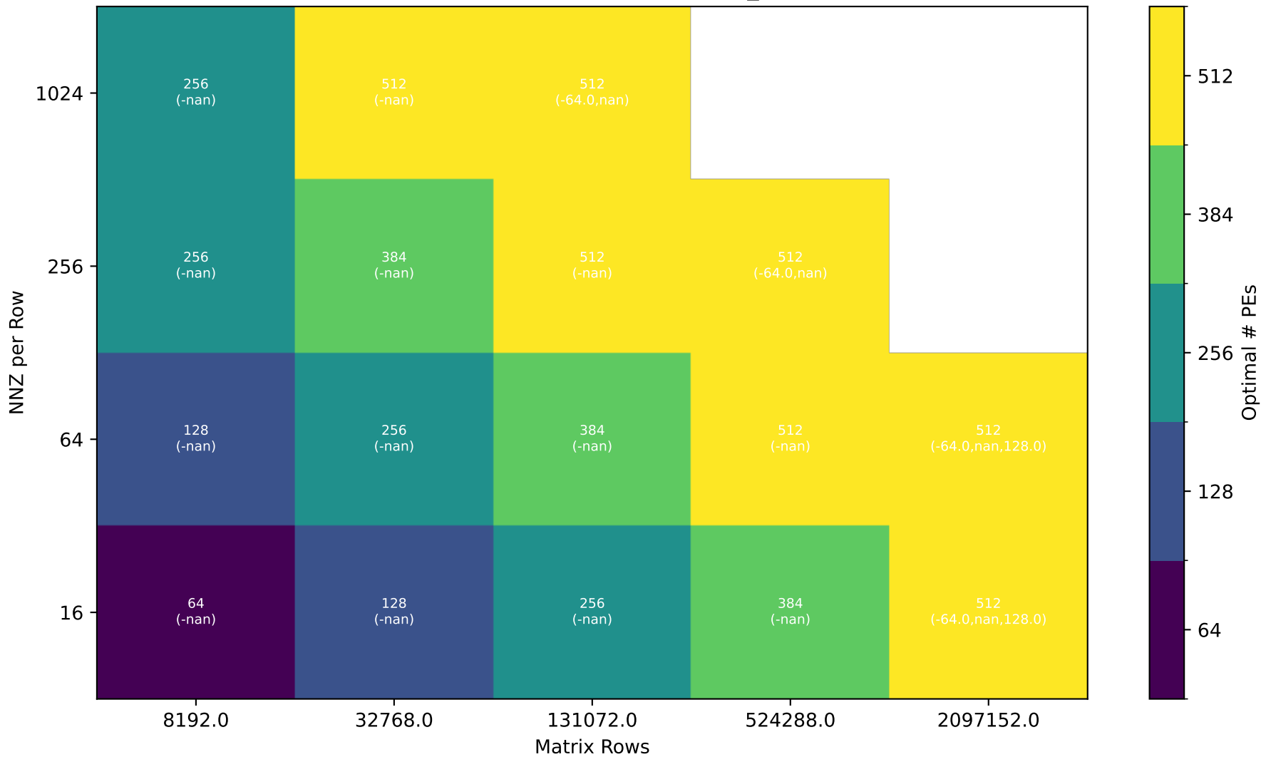
Optimal PE Count (minimum max_time)
