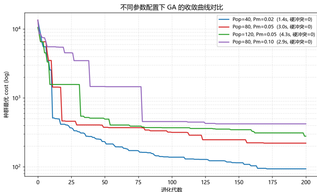
图 6-3 不同参数配置下的收敛曲线对比
