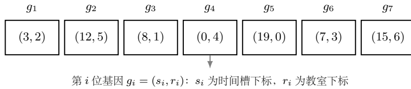
图 4-1 染色体编码示意
