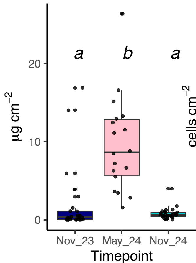
Chl a
