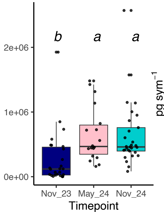
Symbiont density
