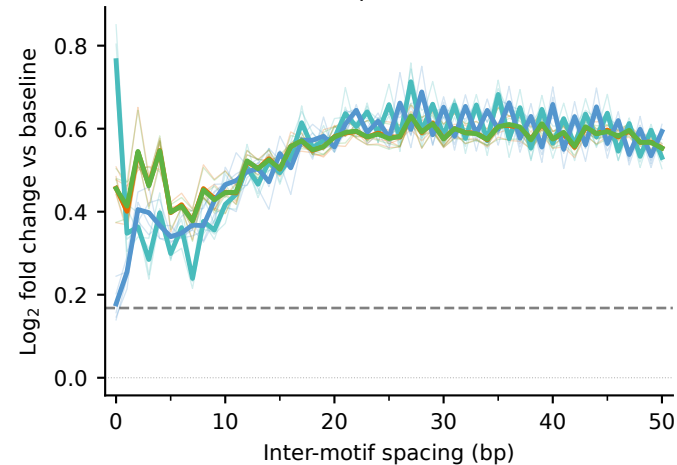
p300
