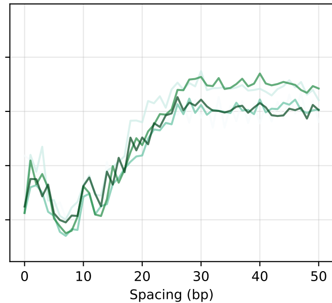
2 motifs, -+
