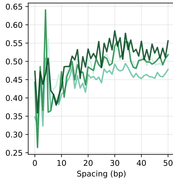
2 motifs, --
