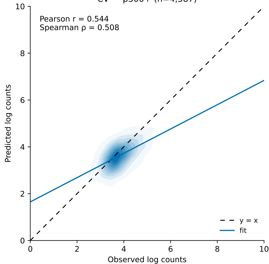
CV — p300+ (n=4,587)
