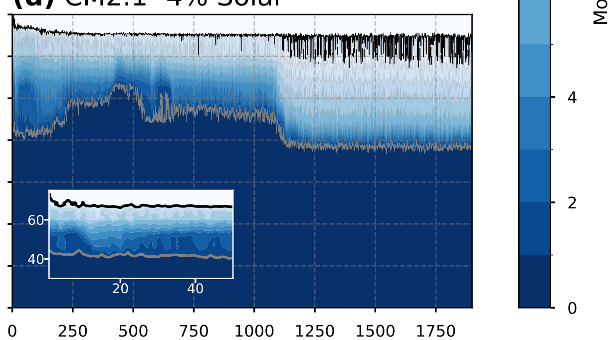
(d) CM2.1 -4% Solar
