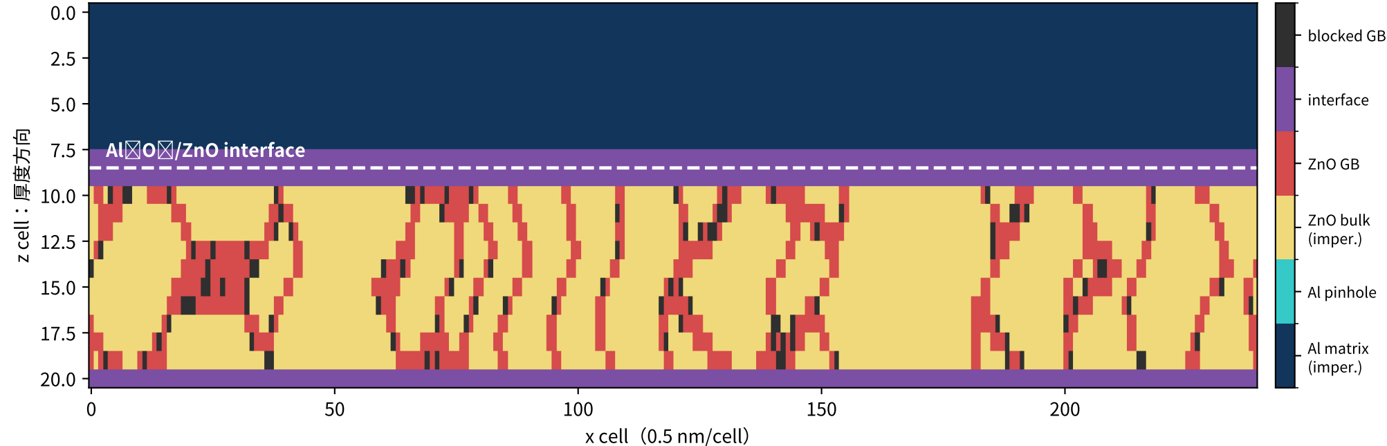
A. 3D 双层结构切片（z-x, y = mid）
