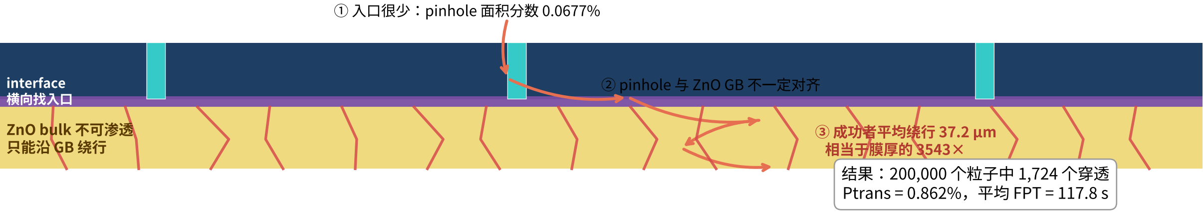
F. 通俗机制：入口少 + 上下层错配 + 晶界绕行，导致低穿透率和高曲折率
