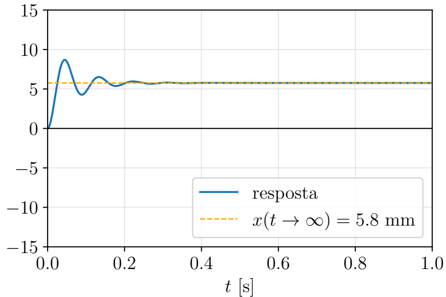
(b) Resposta a funció escaló F(t) = 120 u(t) N
