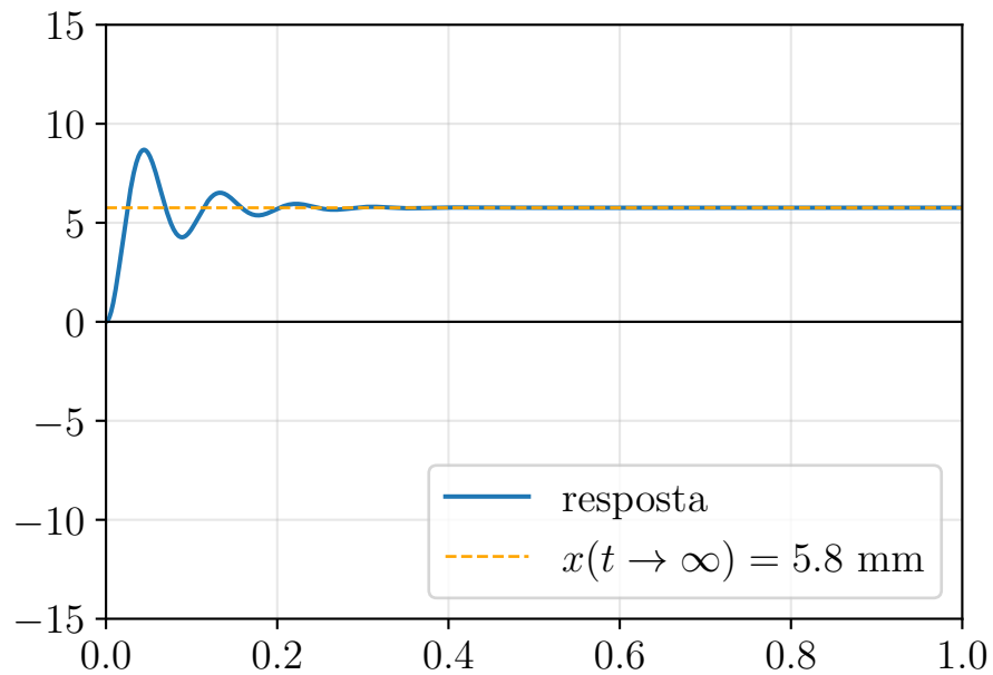
(b) Resposta a funció escalo F(t) = 120 u(t) N
