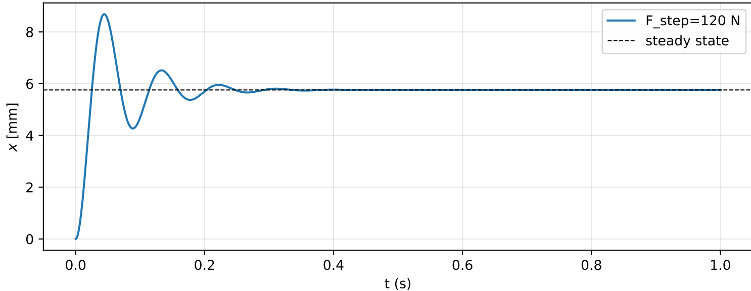
Resposta al pas de força (120 N)
