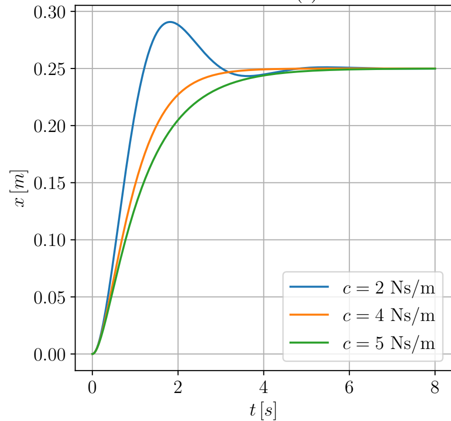
Posició x(t)
