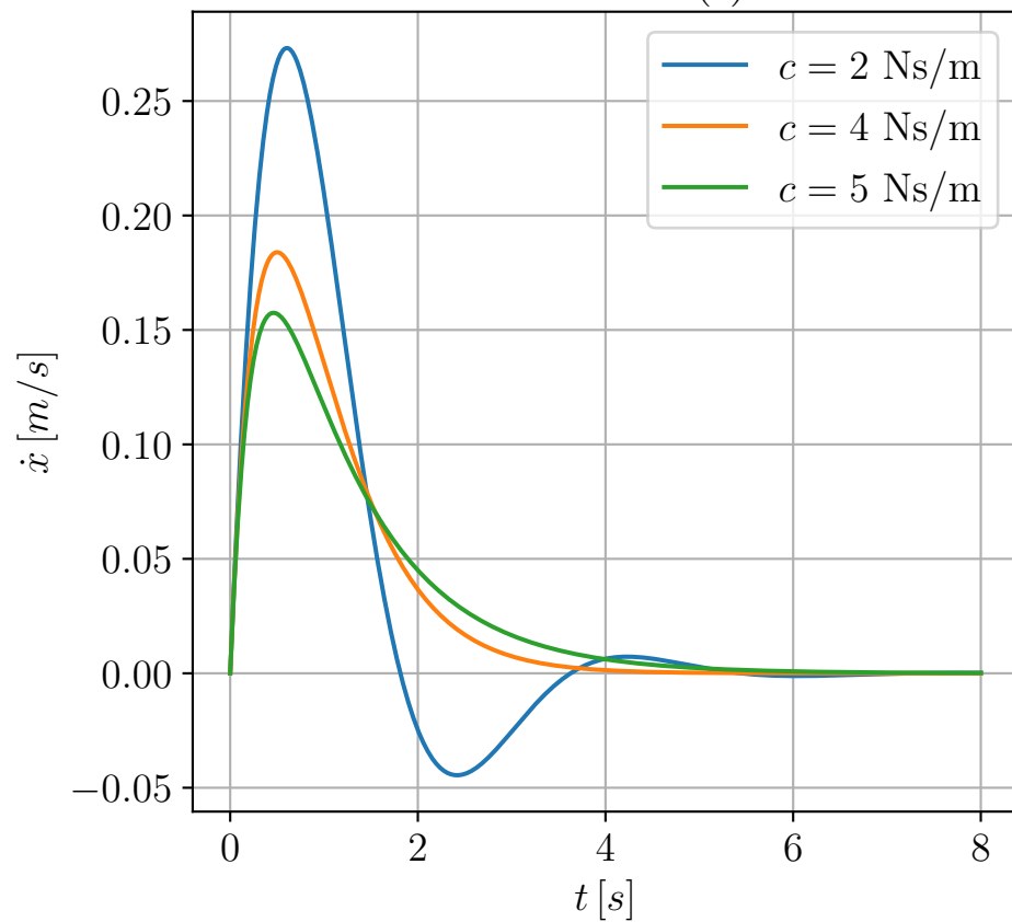
Velocitat \dot{x}(t)
