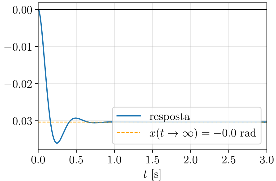
(b) Resposta a funció escaló F(t) = -3.5 u(t) N
