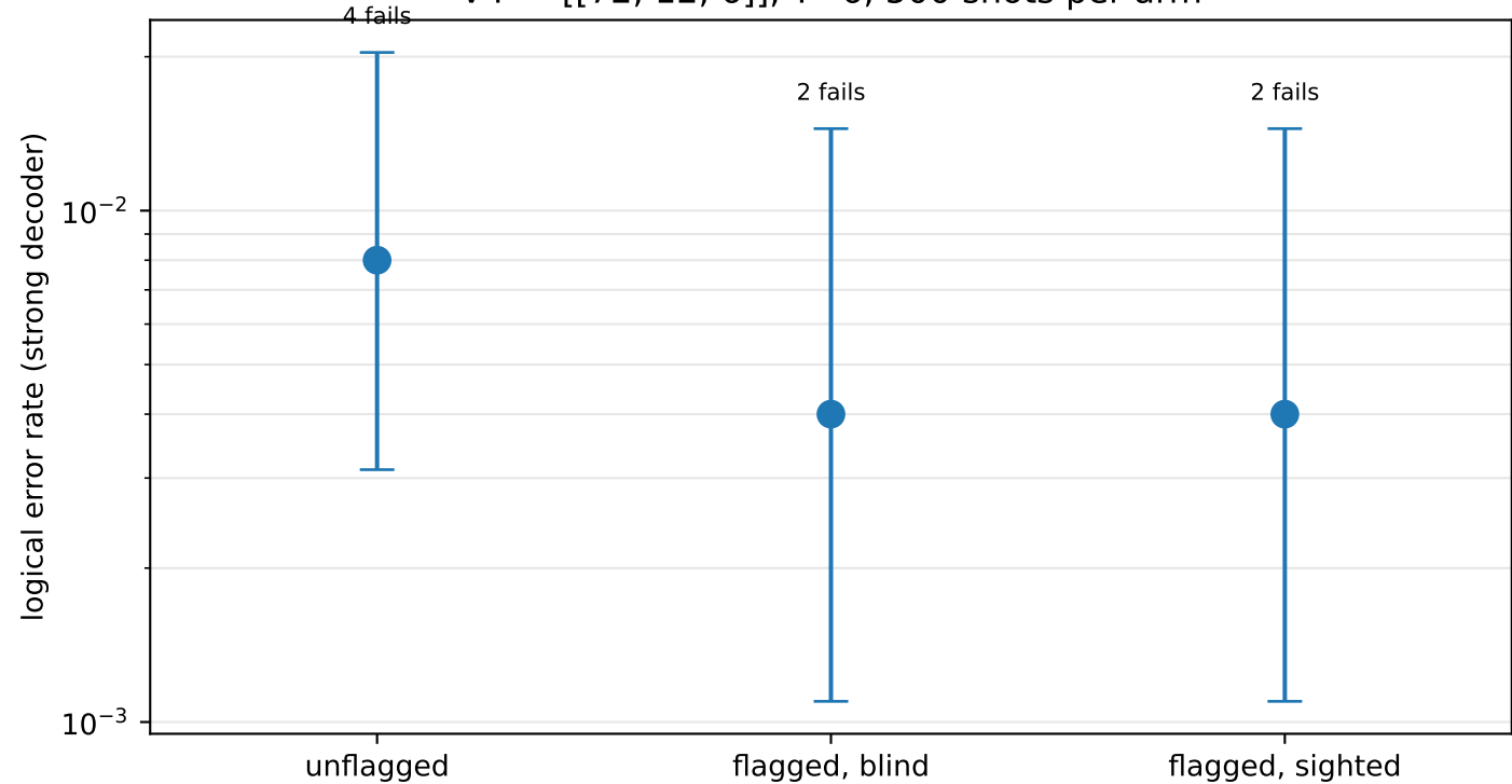
V4 — [[72, 12, 6]] , T=6 , 500 shots per arm
