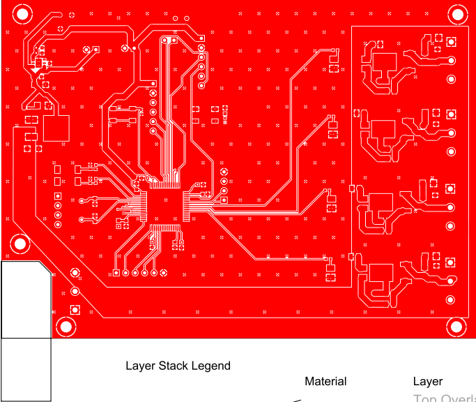
Top Layer (Scale 1:1)
