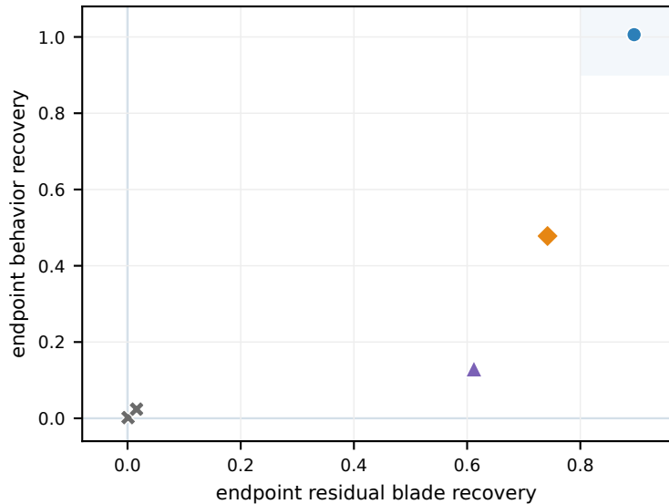
70B
