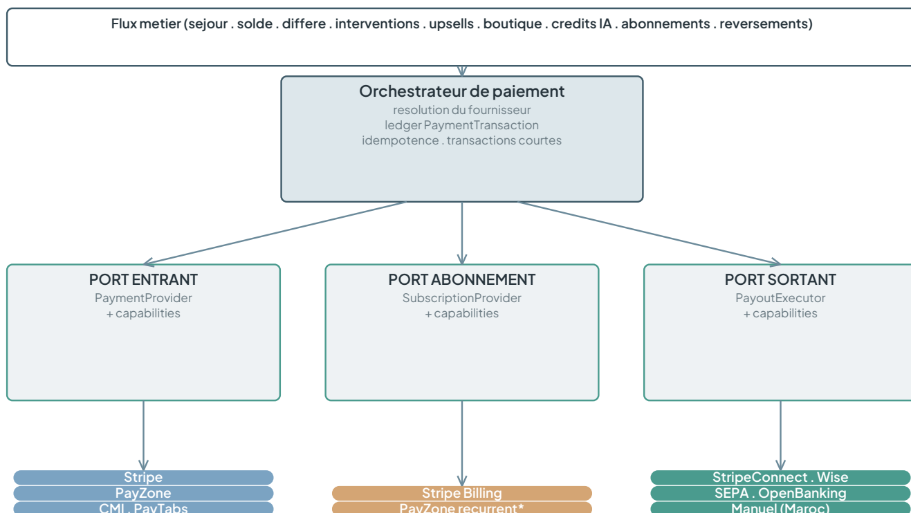
Figure 1 — Architecture hexagonale : un orchestrateur central, trois ports (entrant, abonnement, sortant), des adaptateurs interchangeables. * = à venir.
