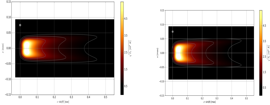
(c) Mapa de temperatura de brillo en el cielo, R_{out,0} = 135R_g R_{in,0} = 100R_g (d) Mapa de temperatura de brillo en el cielo, R_{out,0} = 135R_g R_{in,0} = 130R_g
