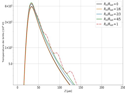
(a) Perfil de brillo superficial logarítmico para distintos valores de R_{in,0} . Fijamos el valor de R_{out,0} = 150 R_g .
