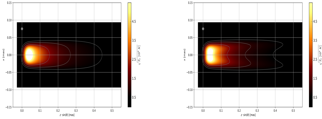
(a) Mapa de temperatura de brillo en el cielo, R_{in,0} = 0 (b) Mapa de temperatura de brillo en el cielo, R_{out,0} = 135R_g R_{in,0} = 75R_g
