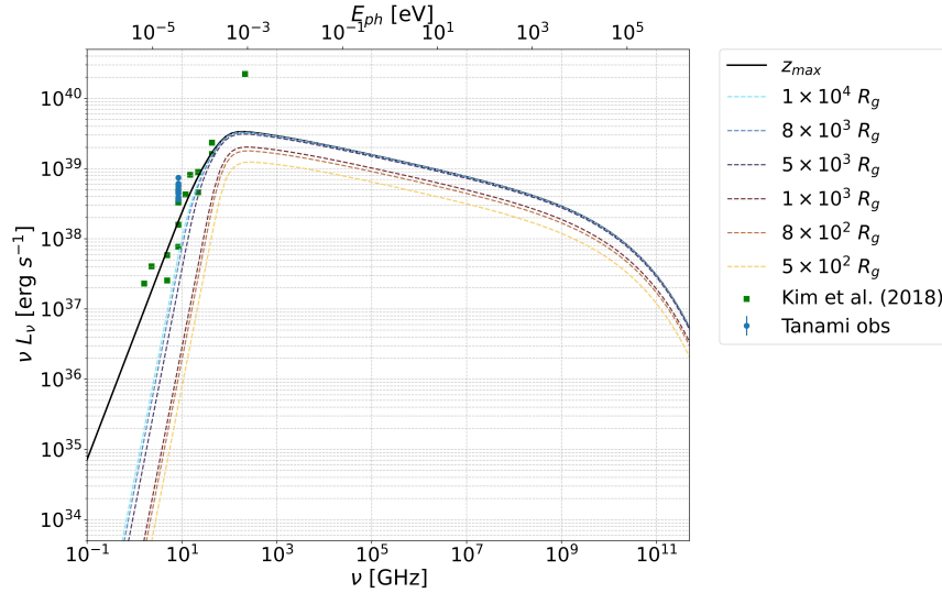
Figura 4.7. Flujo integrado hasta distintas alturas a lo largo del jet , en función de la frecuencia. La curva negra ilustra la emisión integrada sobre toda la altura del jet . En verde se muestran las observaciones compiladas por Kim et al. (2018); en azul las observaciones por Müller et al. (2014). Todavía tengo que ver el tema de EHT
