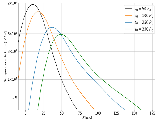
(b) Perfil de brillo superficial logarítmico para valores de z_0 entre 50 R_g y 350 R_g .
