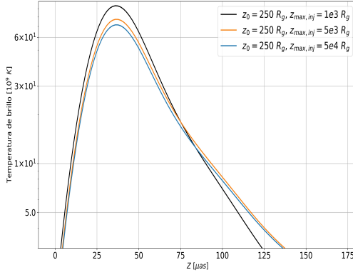
(c) Perfil de brillo superficial logarítmico para distintos valores de z_{max,inj} . Fijamos el valor de z_0 = 250 R_g .
