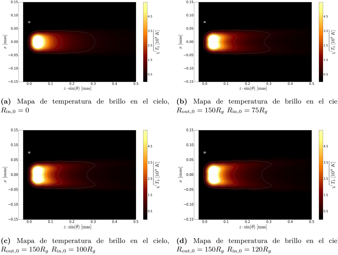
Figura 4.2. Mapas de temperatura de brillo para diversos valores de R_{out,0} , R_{in,0}
