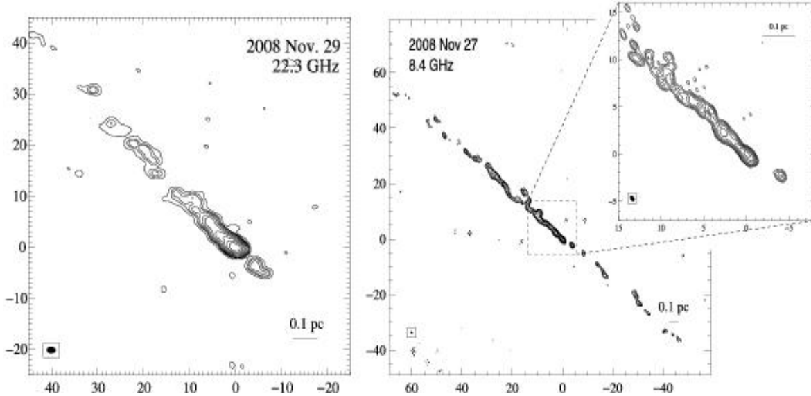
Figura 2.3. Mapas de contorno de Cen A obtenido por el programa de monitoreo TANAMI en frecuencias de 8.4 GHz y 22.3 GHz (Müller et al., 2011)
