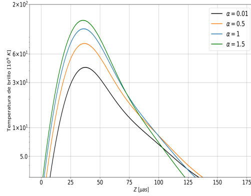
(d) Perfil de brillo superficial logarítmico para distintos valores de a_{inj}
