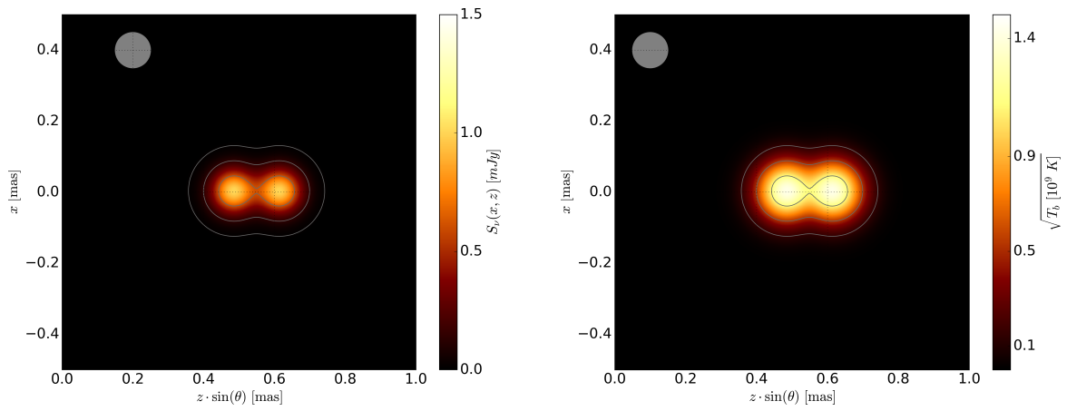
(a) Mapa de prueba de flujo para dos fuentes puntuales proyectado en coordenadas x y z en el plano del cielo.
