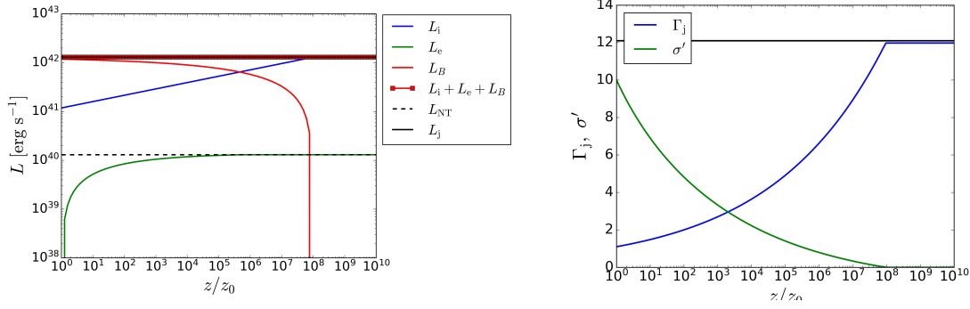
(a) Figura ilustrativa del balance en las componentes (b) Figura ilustrativa de la evolución de la magnetización y el factor de Lorentz a lo largo del jet .
