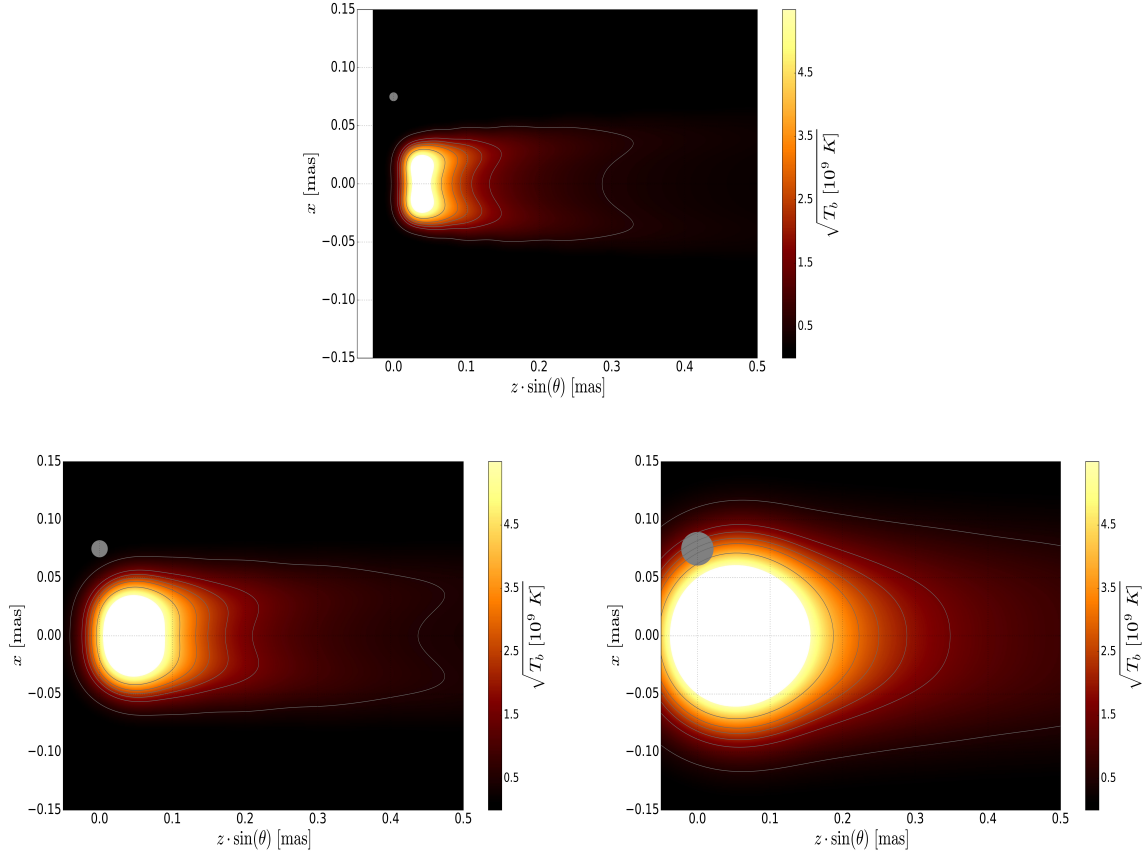
Figura 4.3. Mapas de temperatura de brillo para diversos haces gaussianos de convolución. El haz utilizado para la convolución se encuentra representado por la elipse gris en la esquina superior izquierda de cada mapa. Figura superior: Se utiliza un haz gaussiano con valores de FWHM 0.0168 mas y 0.0259 mas para x, y respectivamente. Figura izquierda: Se utiliza un haz gaussiano con valores de FWHM 2 veces los de la figura superior. Figura derecha: Se utiliza un haz gaussiano con valores de FWHM 4 veces los de la figura superior.
