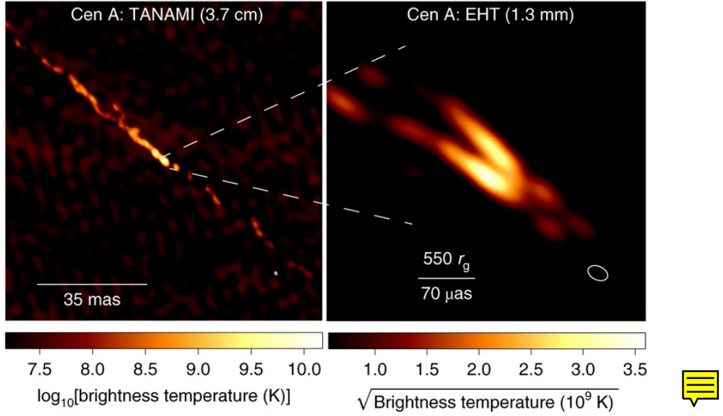
Figura 2.4. Estructura del jet de Cen A. Izq. Imagen obtenida del monitoreo TANAMI a una frecuencia de 8.4 GHz. Se muestra la temperatura de brillo en escala logarítmica (Noviembre 2011). Der. Imagen obtenida por el EHT a una frecuencia de 228 GHz que revela estructuras a una escala mucho más pequeña. La escala de colores corresponde a la raíz cuadrada de la temperatura de brillo (Abril 2017). (Janssen et al., 2021)
