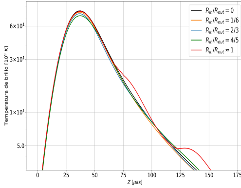
(a) Perfil de brillo superficial logarítmico para distintos valores de R_{in,0} . Fijamos el valor de R_{out,0} = 150 R_g .
