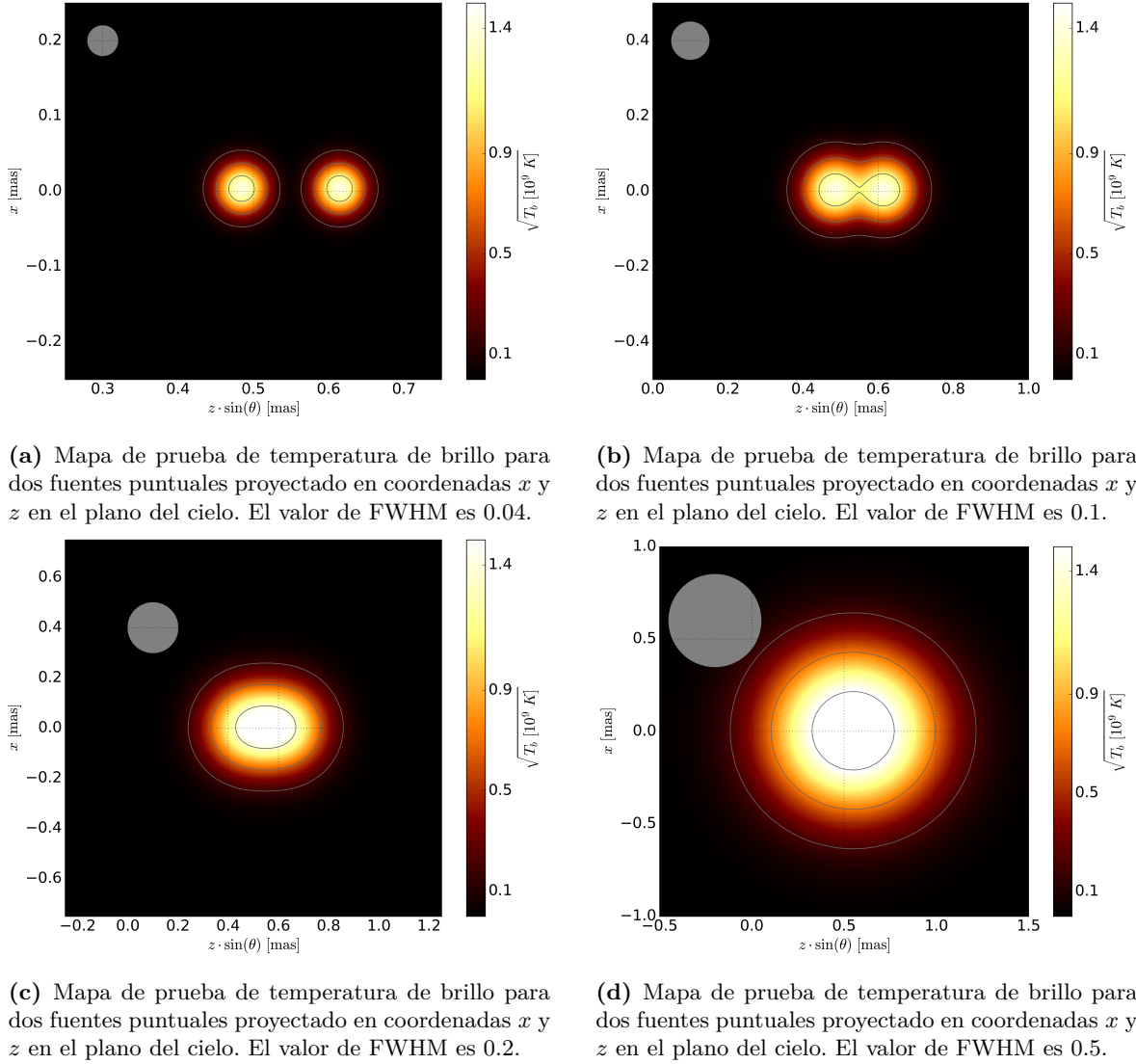
Figura 3.7. Prueba de convolución sobre dos fuentes puntuales para diversos valores de FWHM.
