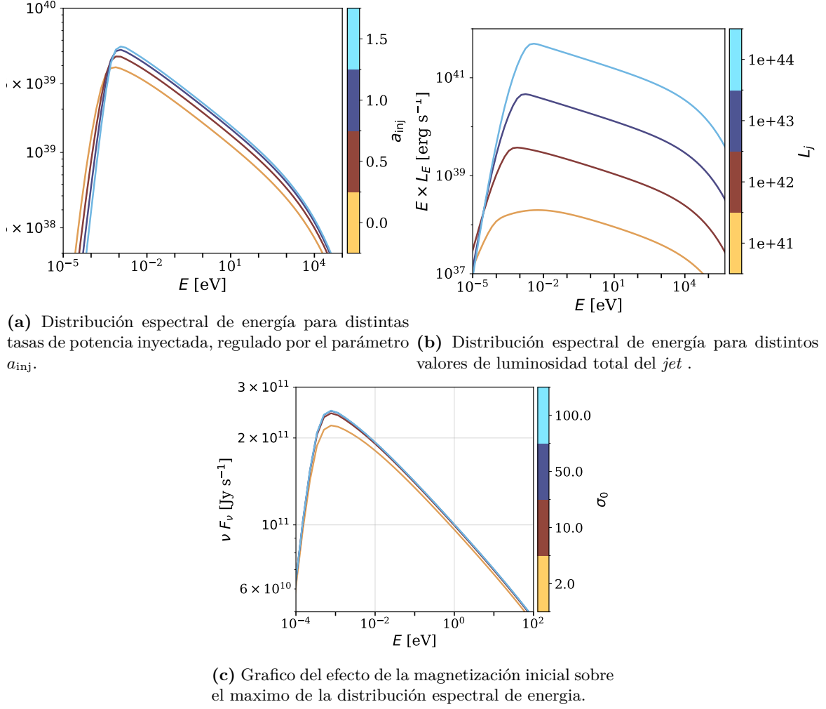
Figura 4.1. Exploración de parámetros a_{\text{inj}} , L_j y \sigma_0 para los gráficos de distribución espectral de energía (Fig. a,b ) y para el maximo de la misma (Fig. c ).
