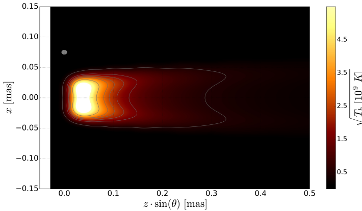
Figura 4.9. Mapa de temperatura de brillo proyectado en coordenadas x y z en el plano del cielo, obtenido a partir del ajuste al modelo para las observaciones de Cen A. El suavizado se realizó mediante un haz gaussiano con anchos a media altura (FWHM) de 0.0168 mas en la dirección x y 0.0259 mas en la dirección y .
