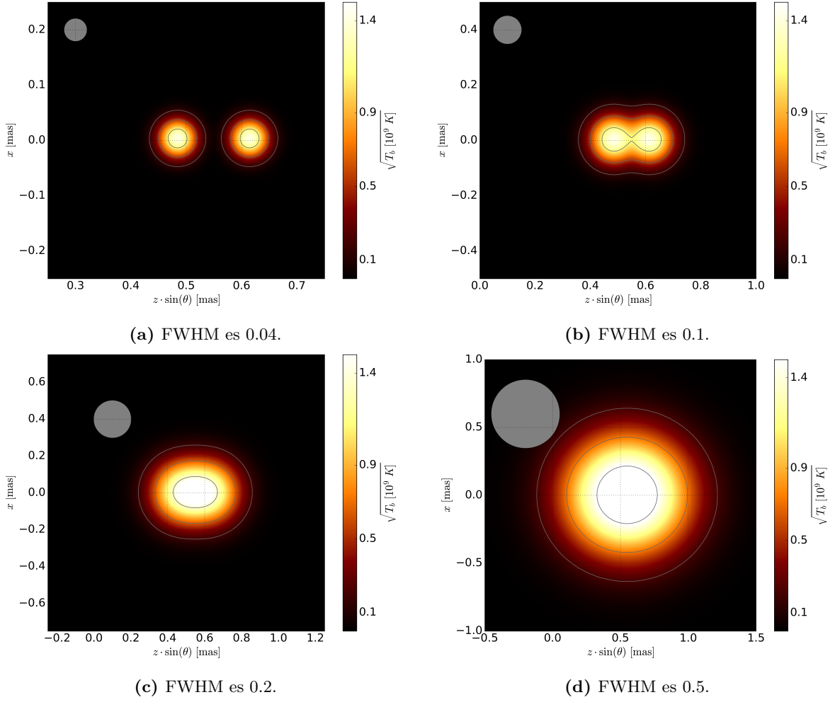
Figura 3.6. Mapa de prueba de temperatura de brillo proyectado en coordenadas x y z en el plano del cielo con valores de FWHM: 0.04 (panel superior izquierdo), 0.1 (panel superior derecho), 0.2 (panel inferior izquierdo), 0.5 (panel inferior derecho).
