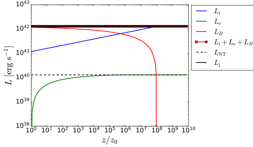
(a) Balance en las componentes de la potencia a lo largo del jet .
