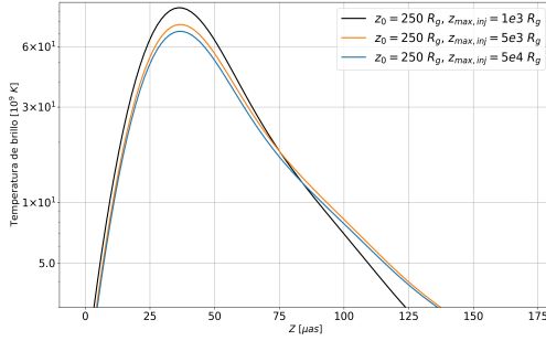
(c) z_{max,inj} . Fijamos el valor de z_0 = 250 R_g .
