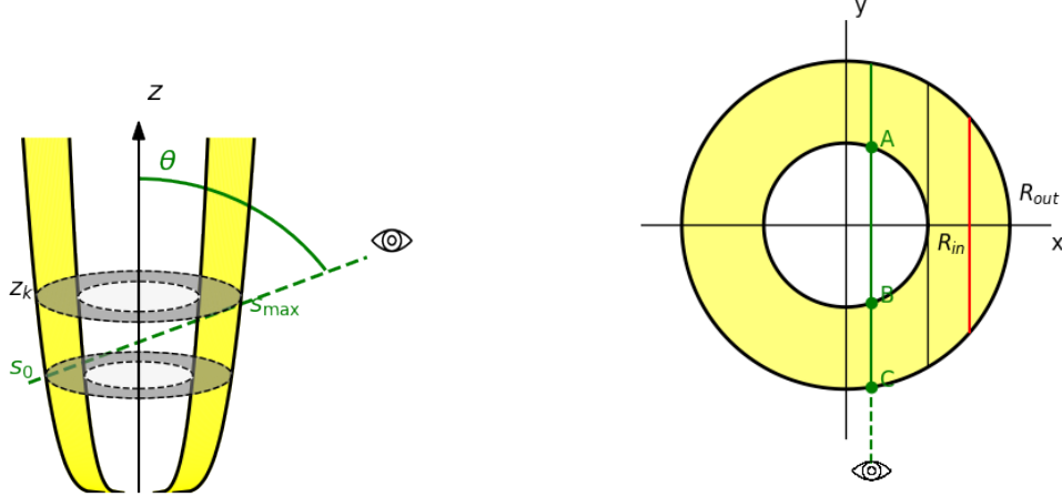
(a) Diagrama del cruce de un rayo de luz por el espesor del jet .
