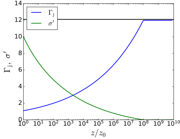
(b) Evolución de la magnetización y el factor de Lorentz a lo largo del jet
