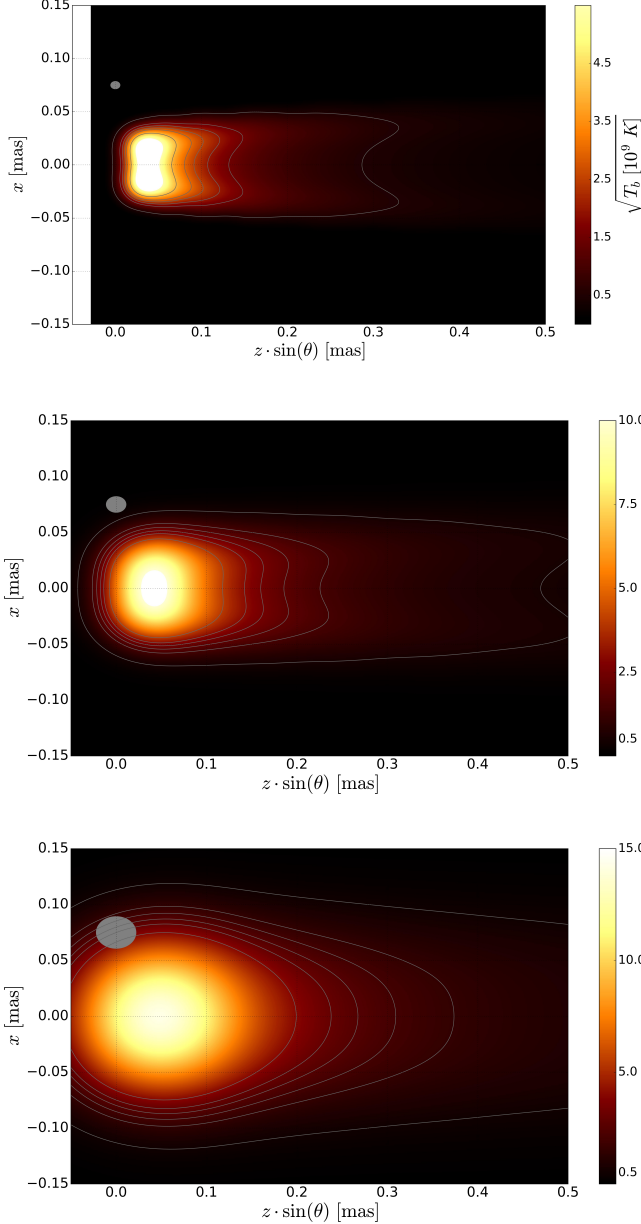
Figura 4.4. Mapas de temperatura de brillo para diversos haces gaussianos de convolución. El haz utilizado para la convolución se encuentra representado por la elipse gris en la esquina superior izquierda de cada mapa.
