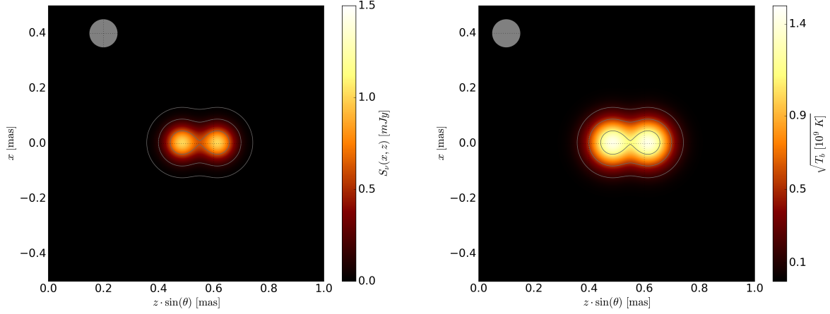
Figura 3.5. Resultados de la convolución sobre dos fuentes puntuales de igual flujo con un haz gaussiano de \text{FWHM} = 0.1 mas. Mapa de flujo (panel izquierdo) y temperatura de brillo (panel derecho) proyectados en coordenadas x y z en el plano del cielo.
