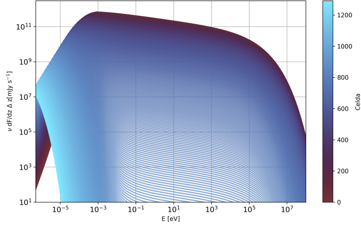
Figura 4.7. Flujo emitido por cada una de las 1293 celdas en las que se subdivide el jet . El jet se divide en celdas de altura \Delta z . Modelamos individualmente la emisión en cada una de estas.
