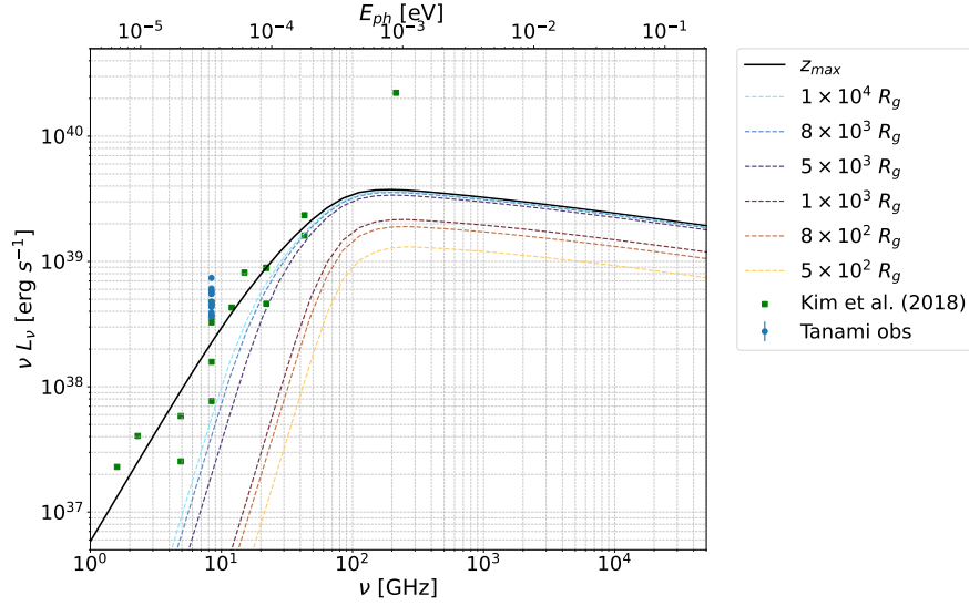
Figura 4.8. Flujo integrado hasta distintas alturas a lo largo del jet , en función de la frecuencia. La curva negra ilustra la emisión integrada sobre toda la altura del jet . En verde se muestran las observaciones compiladas por Kim et al. (2018); en azul las observaciones por Müller et al. (2014). Todavía tengo que ver el tema de EHT
