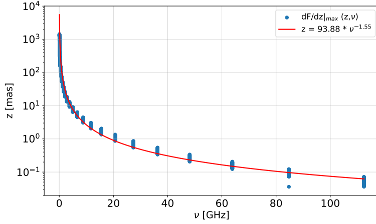
Figura 4.9. Desplazamiento de la frecuencia correspondiente al máximo de emisión a distintas alturas del jet . La figura muestra como la frecuencia correspondiente al máximo de emisión resulta menor a medida que integramos hasta alturas mayores respecto de la base del jet . En rojo presentamos una ley de potencias ajustada a los puntos.
