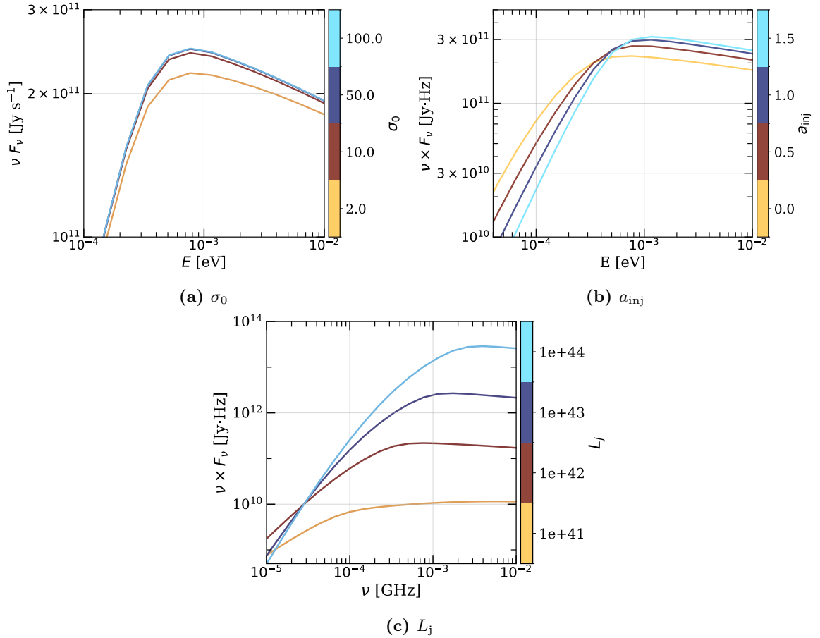
Figura 4.2. Graficos de la distribución espectral de energía en el rango de longitud de onda de radio. Presentamos la exploración de parámetros de \sigma_0 , a_{\text{inj}} y L_j .
