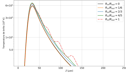
(a) Perfil de brillo superficial logarítmico para distintos valores de R_{in,0} . Fijamos el valor de R_{out,0} = 150 R_g .
