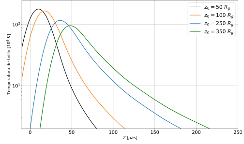
(b) Perfil de brillo superficial logarítmico para valores de z_0 entre 50 R_g y 350 R_g .
