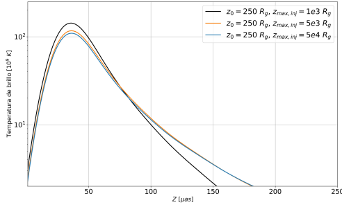
(c) Perfil de brillo superficial logarítmico para distintos valores de z_{max,inj} . Fijamos el valor de z_0 = 250 R_g .
