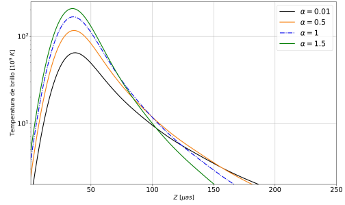
(d) Perfil de brillo superficial logarítmico para distintos valores de a_{inj}
