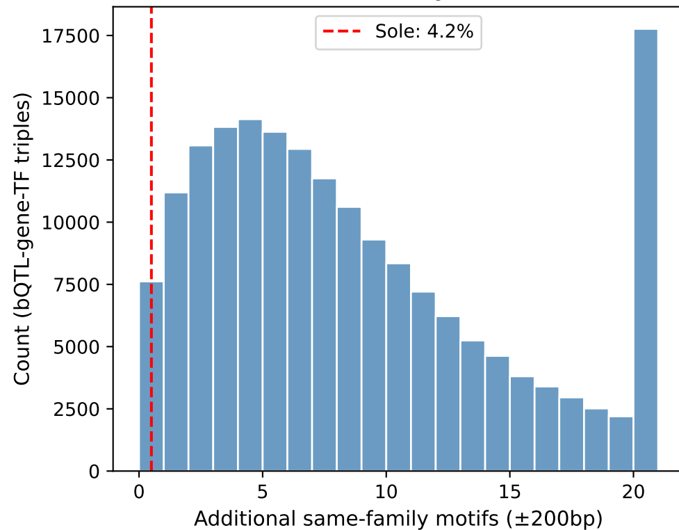
A. Motif redundancy distribution
