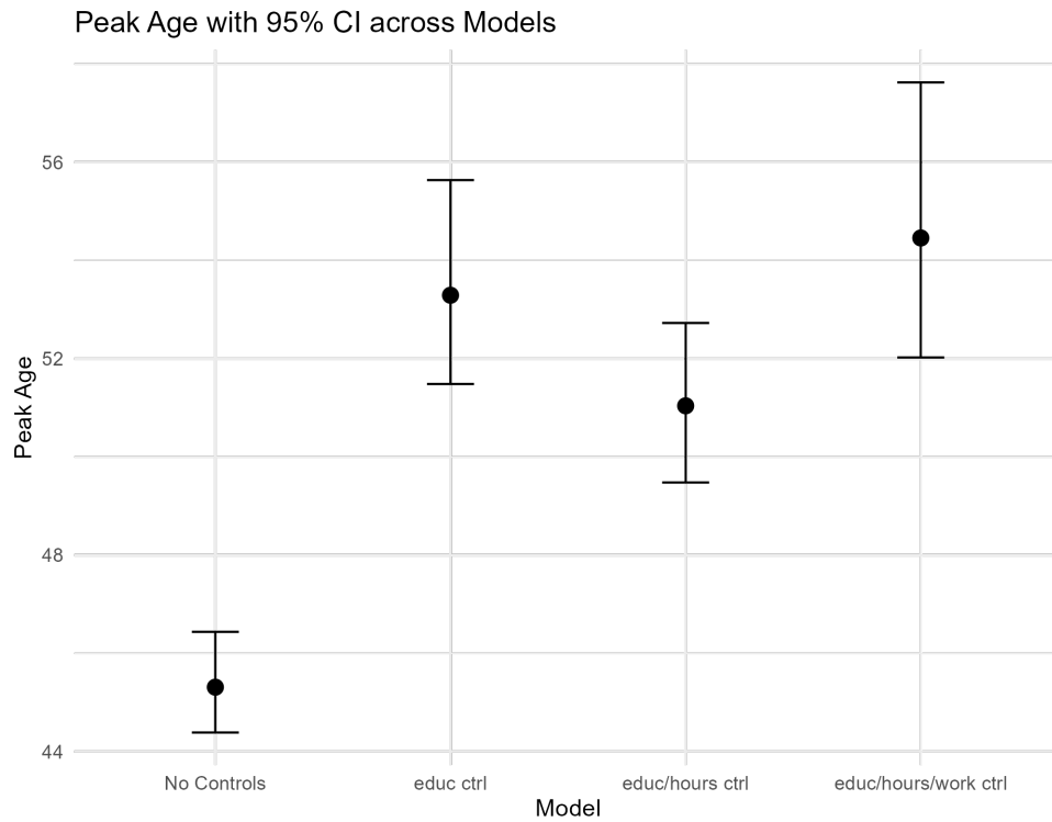
Figura 4. Intervalos de confianza de la edad pico
