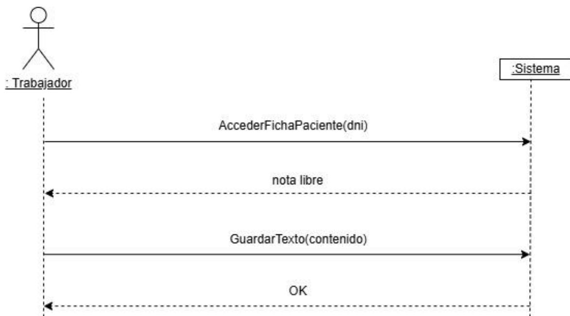
Figura 10: Diagrama de Secuencia del Sistema para el CU-09.
