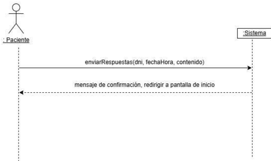
Figura 15: Diagrama de Secuencia del Sistema para el CU-14.
