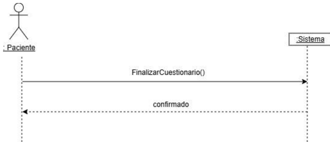
Figura 9: Diagrama de Secuencia del Sistema para el CU-08.
