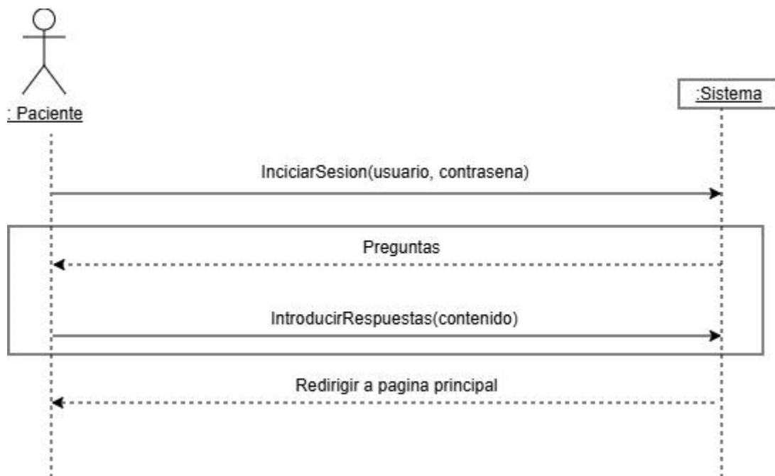
Figura 8: Diagrama de Secuencia del Sistema para el CU-07.
