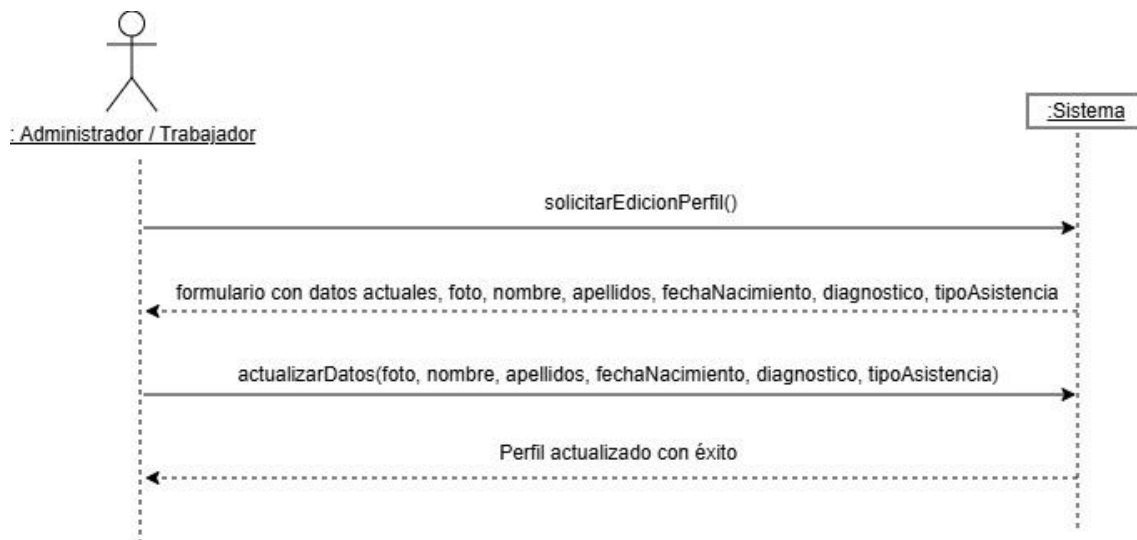
Figura 4: Diagrama de Secuencia del Sistema para el CU-03.
