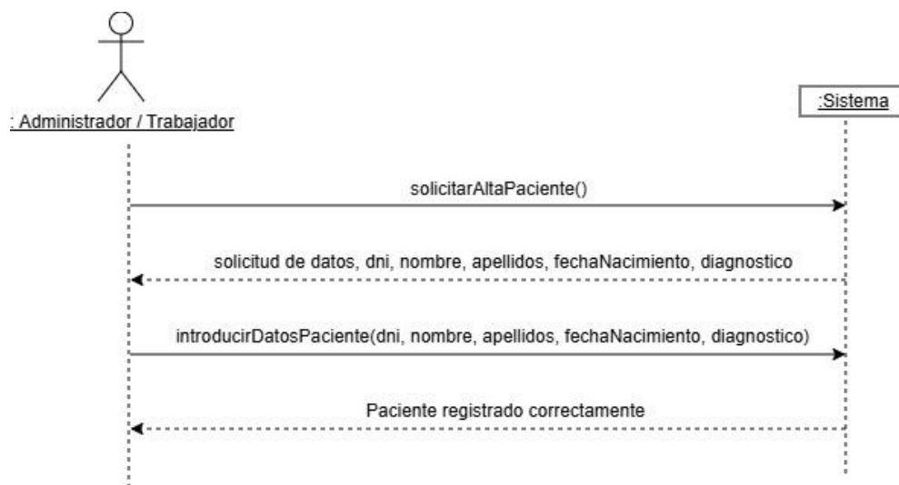
Figura 2: Diagrama de Secuencia del Sistema para el CU-01.
