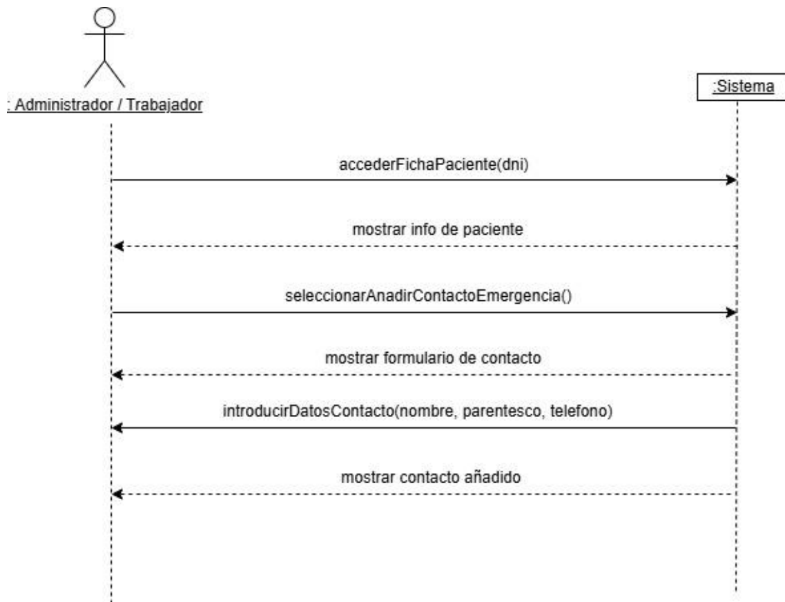
Figura 6: Diagrama de Secuencia del Sistema para el CU-05.
