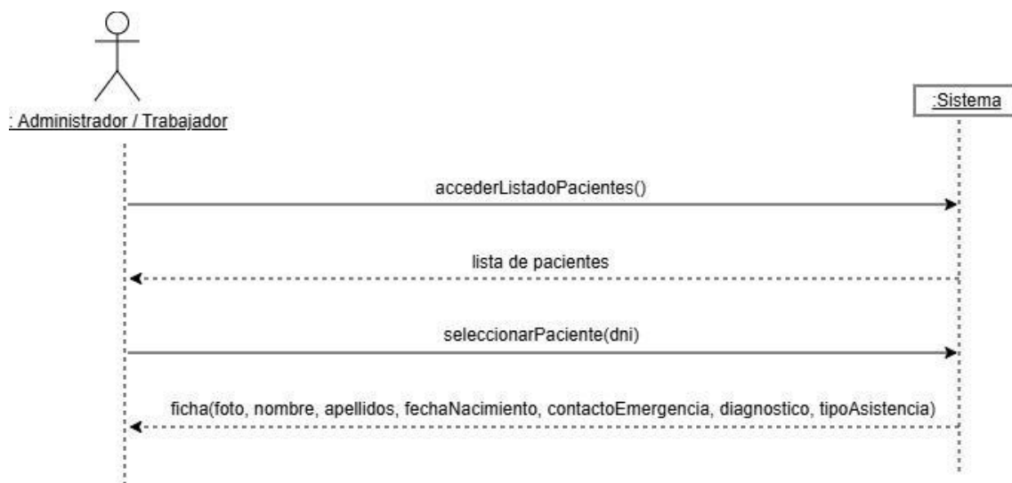
Figura 3: Diagrama de Secuencia del Sistema para el CU-02.
