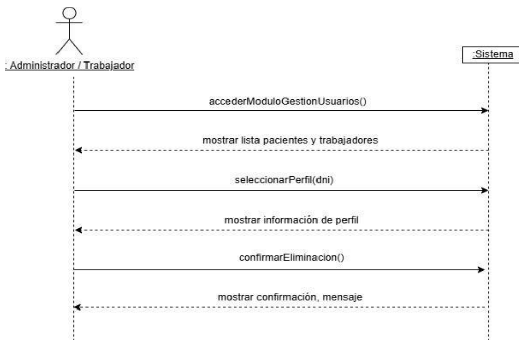
Figura 5: Diagrama de Secuencia del Sistema para el CU-04.
