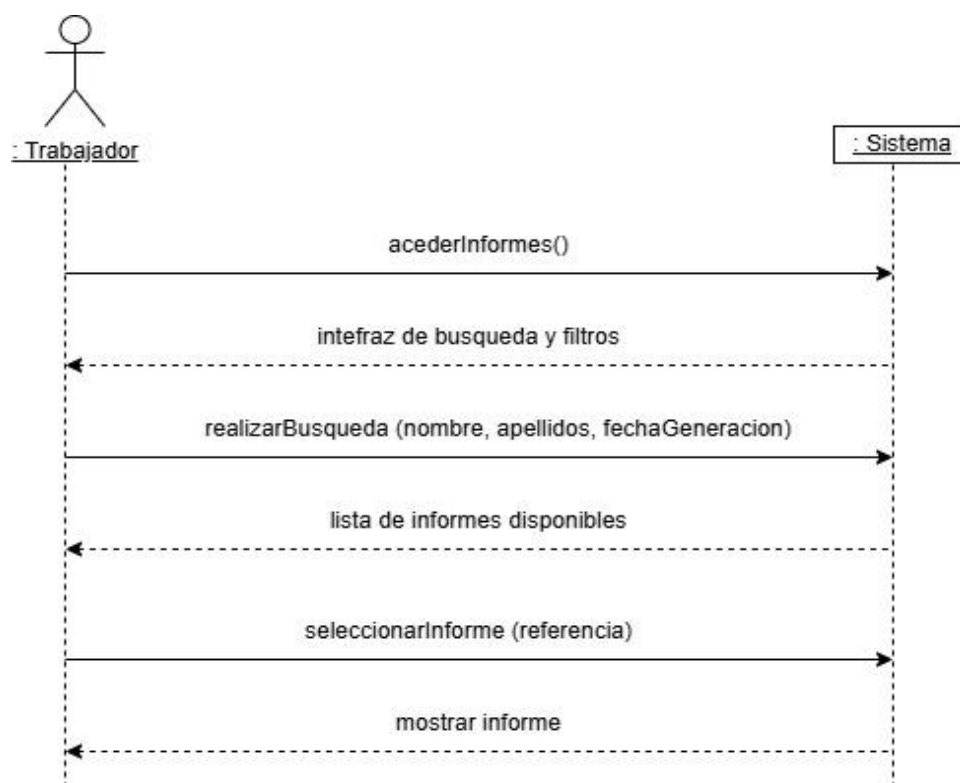
Figura 14: Diagrama de Secuencia del Sistema para el CU-13.
