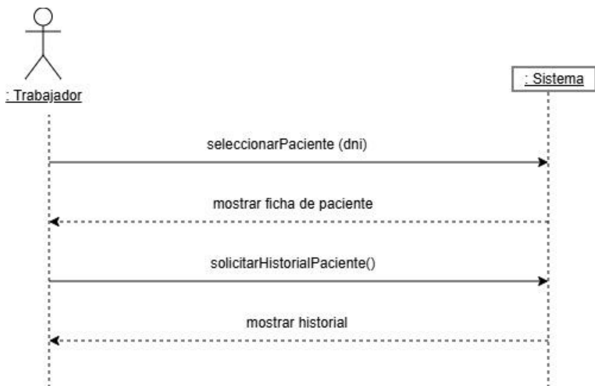
Figura 12: Diagrama de Secuencia del Sistema para el CU-11.
