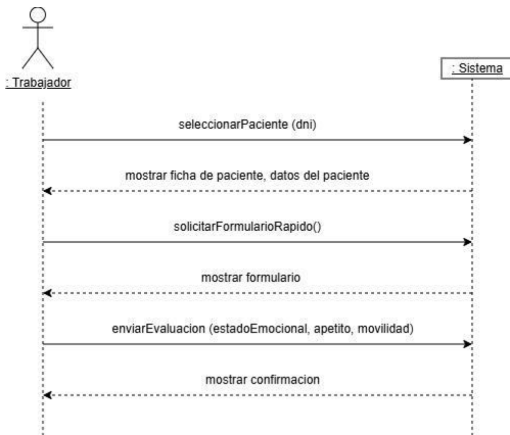
Figura 11: Diagrama de Secuencia del Sistema para el CU-10.
