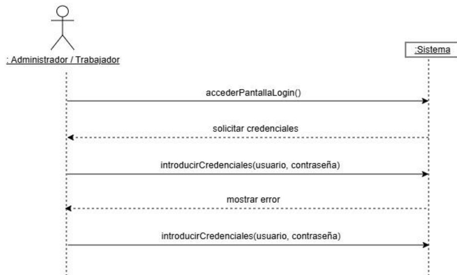
Figura 7: Diagrama de Secuencia del Sistema para el CU-06.
