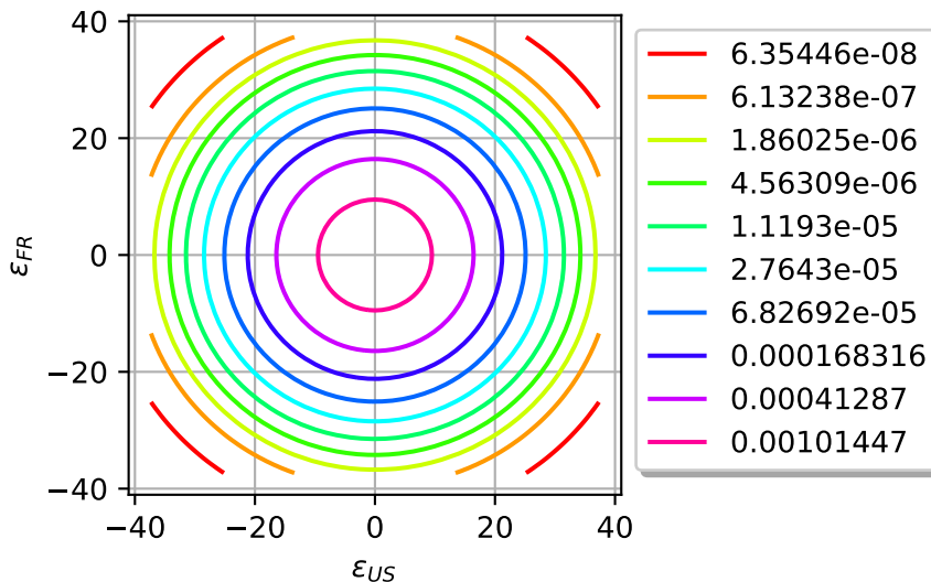
Gaussian Lin.: [ \varepsilon_{US}, \varepsilon_{FR} ] iso-PDF
