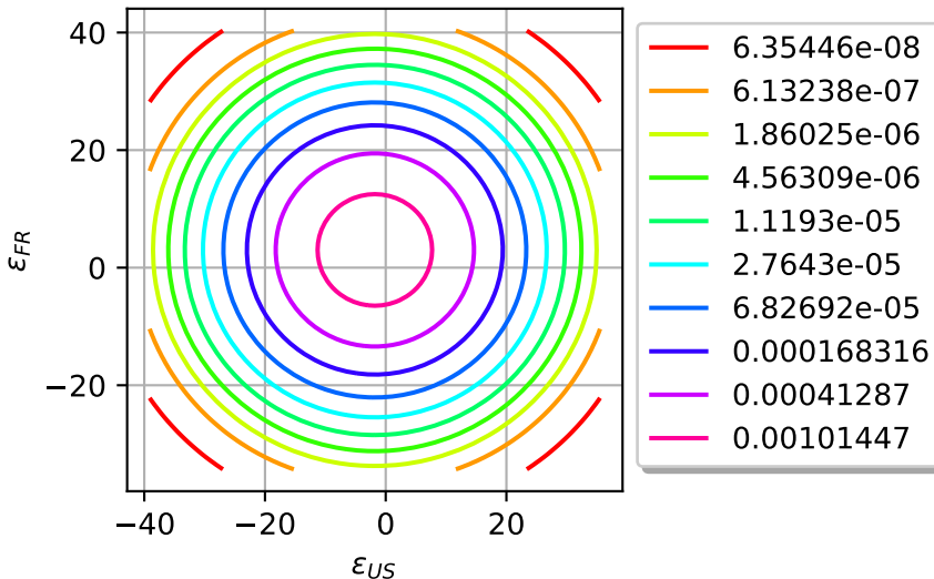
Gaussian N.L.: [ \varepsilon_{US}, \varepsilon_{FR} ] iso-PDF
