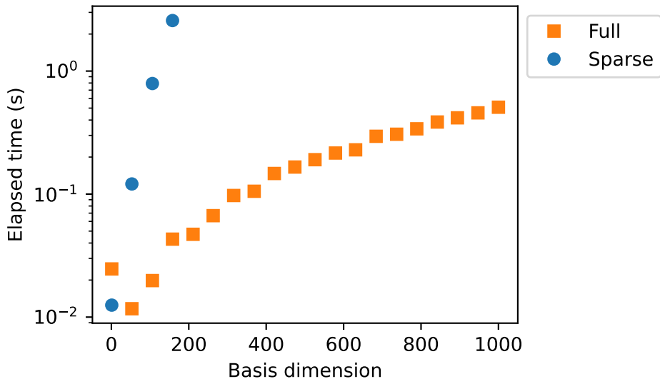
Dirichlet, d=3 , n=1000
