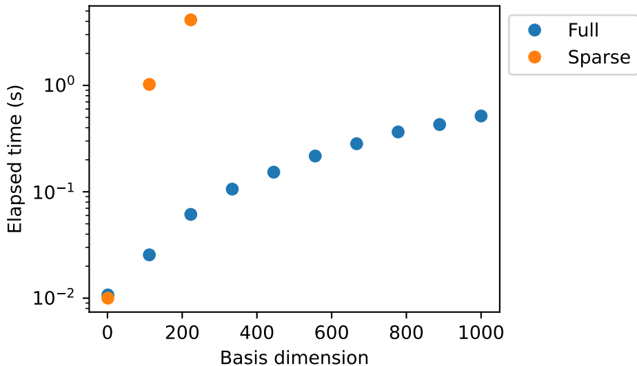
PCE, d=3 , n=1000
