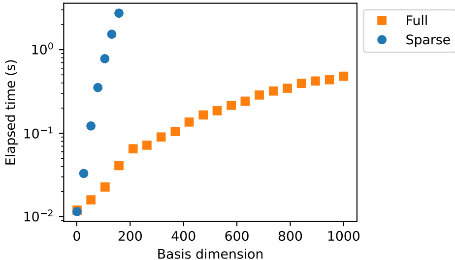
GSobol, d=3 , n=1000
