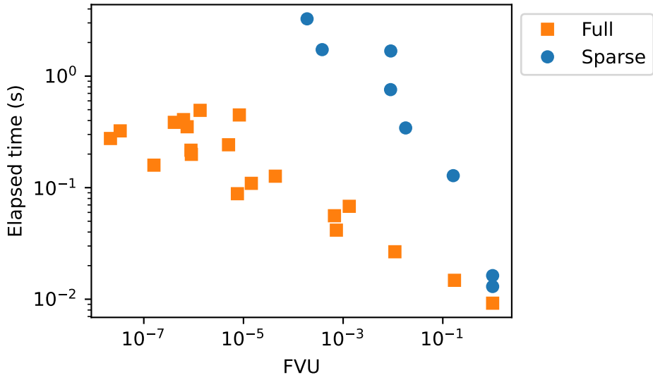
Ishigami, d=3 , n=1000
