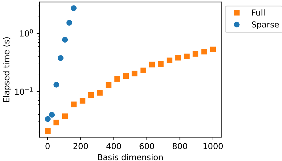
Morris, d=20 , n=1000
