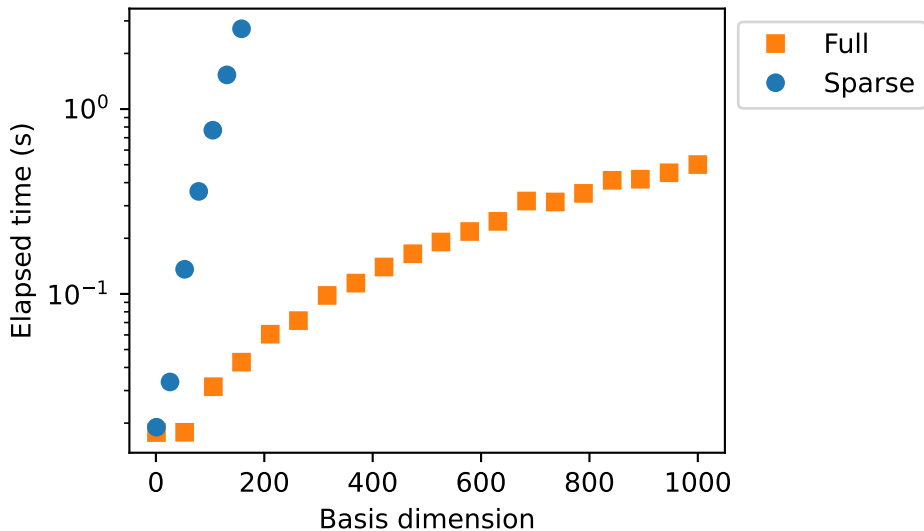
GSobol10, d=10, n=1000
