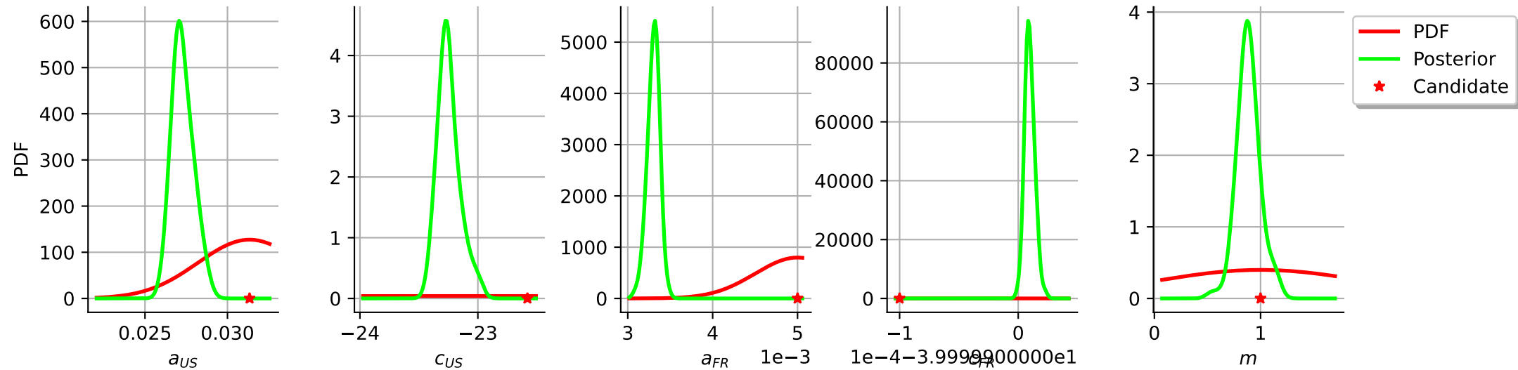
Gaussian N.L.
