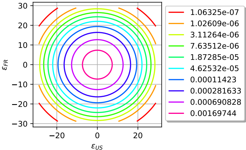
LLS: [\varepsilon_{US}, \varepsilon_{FR}] iso-PDF
