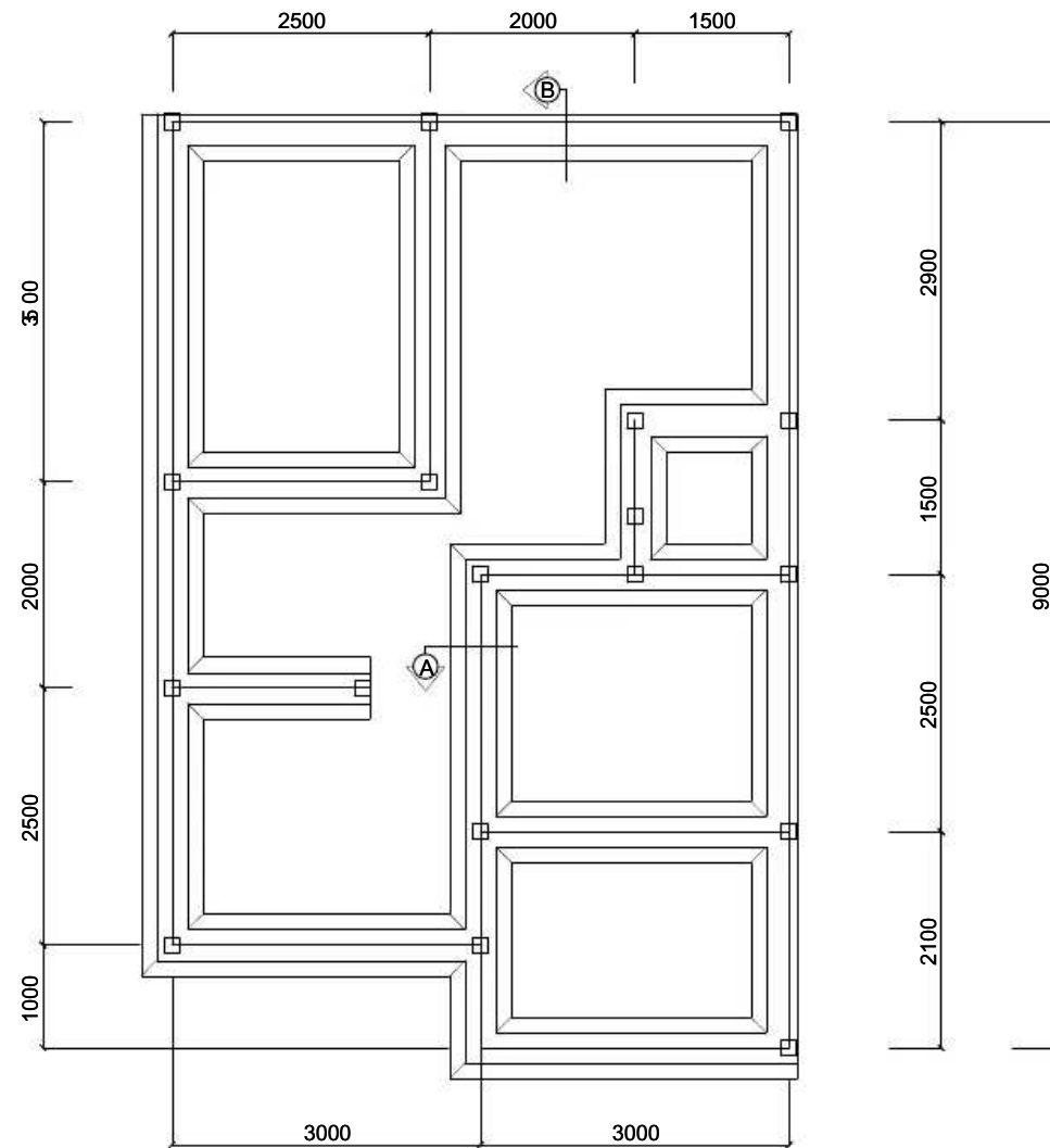
DENAH PONDASI 1:50
