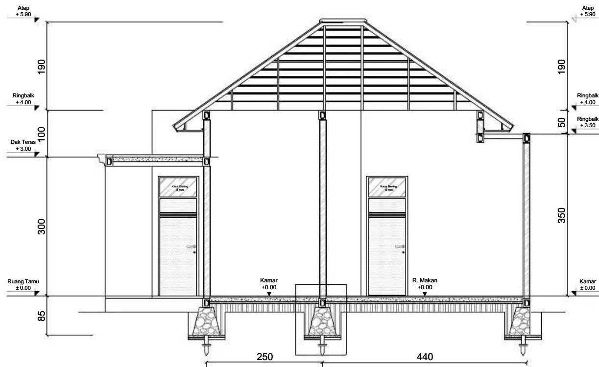
POTONGAN B-B 1:50
