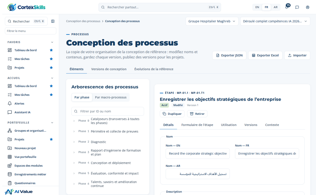
Figure 6 — Conception des processus : arborescence et formulaire de l'élément
