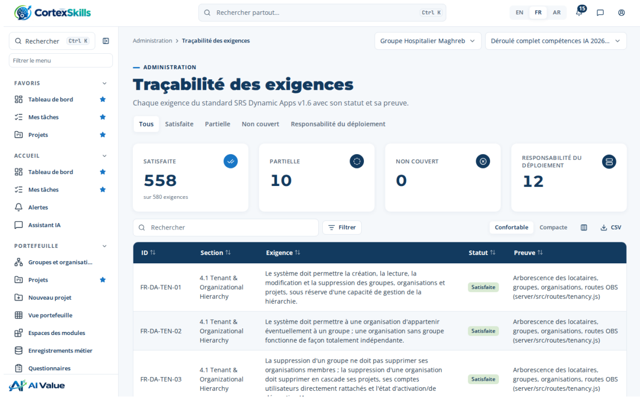
Figure 18 — Traçabilité des exigences
