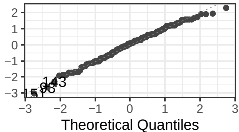
Normal Q-Q
