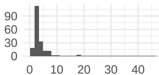
Fe
