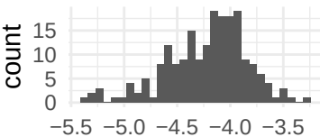
d18O
