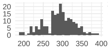
Ca
