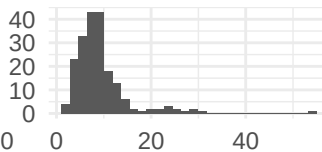
Si
