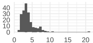
Al
