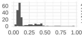
Mn
