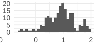
d13C
