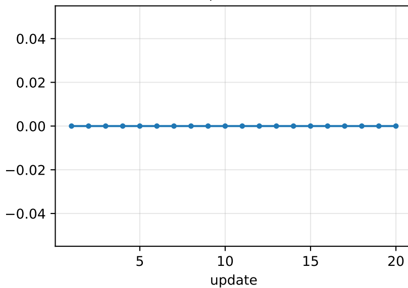
clip fraction
