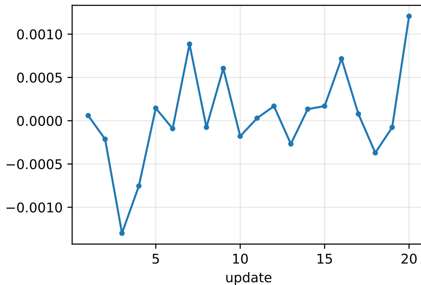
clip fraction
