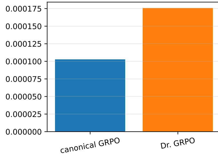
held-out KL
