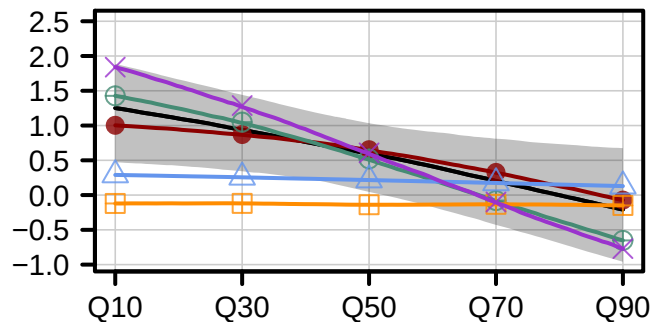
UD ( \eta )
