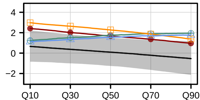
EPL ( \zeta )
