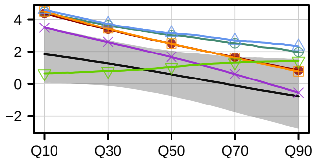
UD ( \eta )
