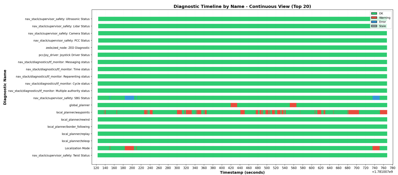
FIGURE 31 – Timeline des diagnostics de l'IHM par nom de diagnostic
