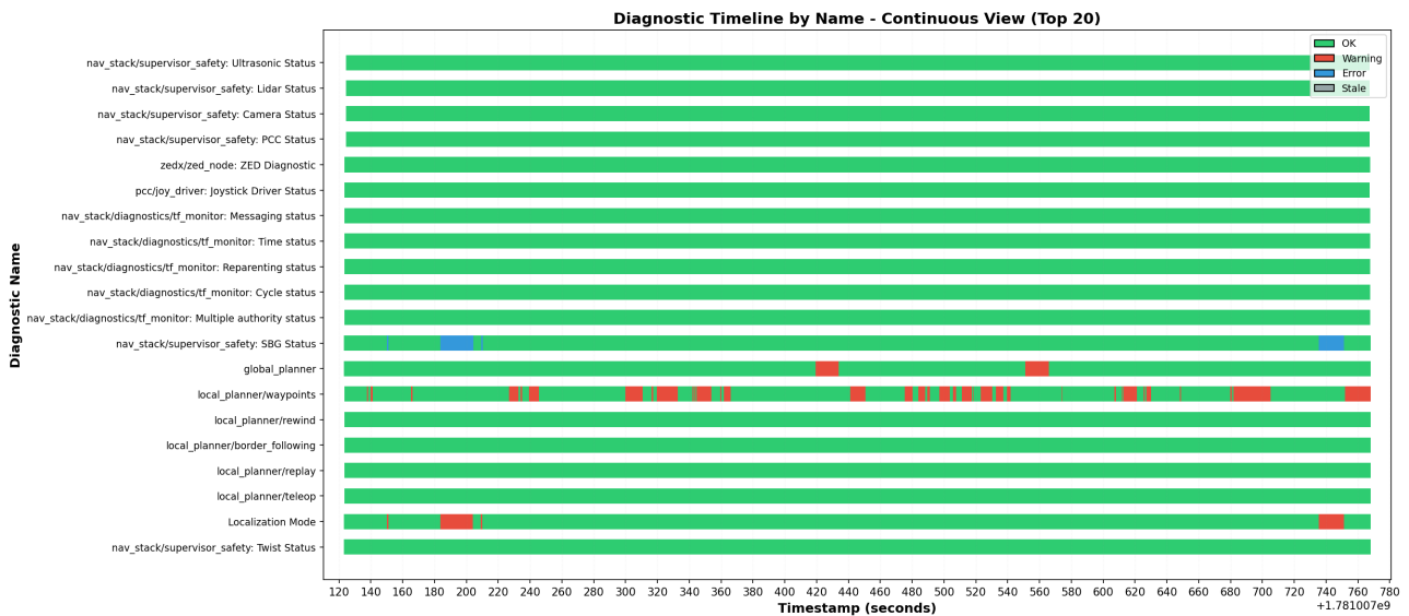
FIGURE 32 – Timeline des diagnostics de l'IHM par nom de diagnostic
